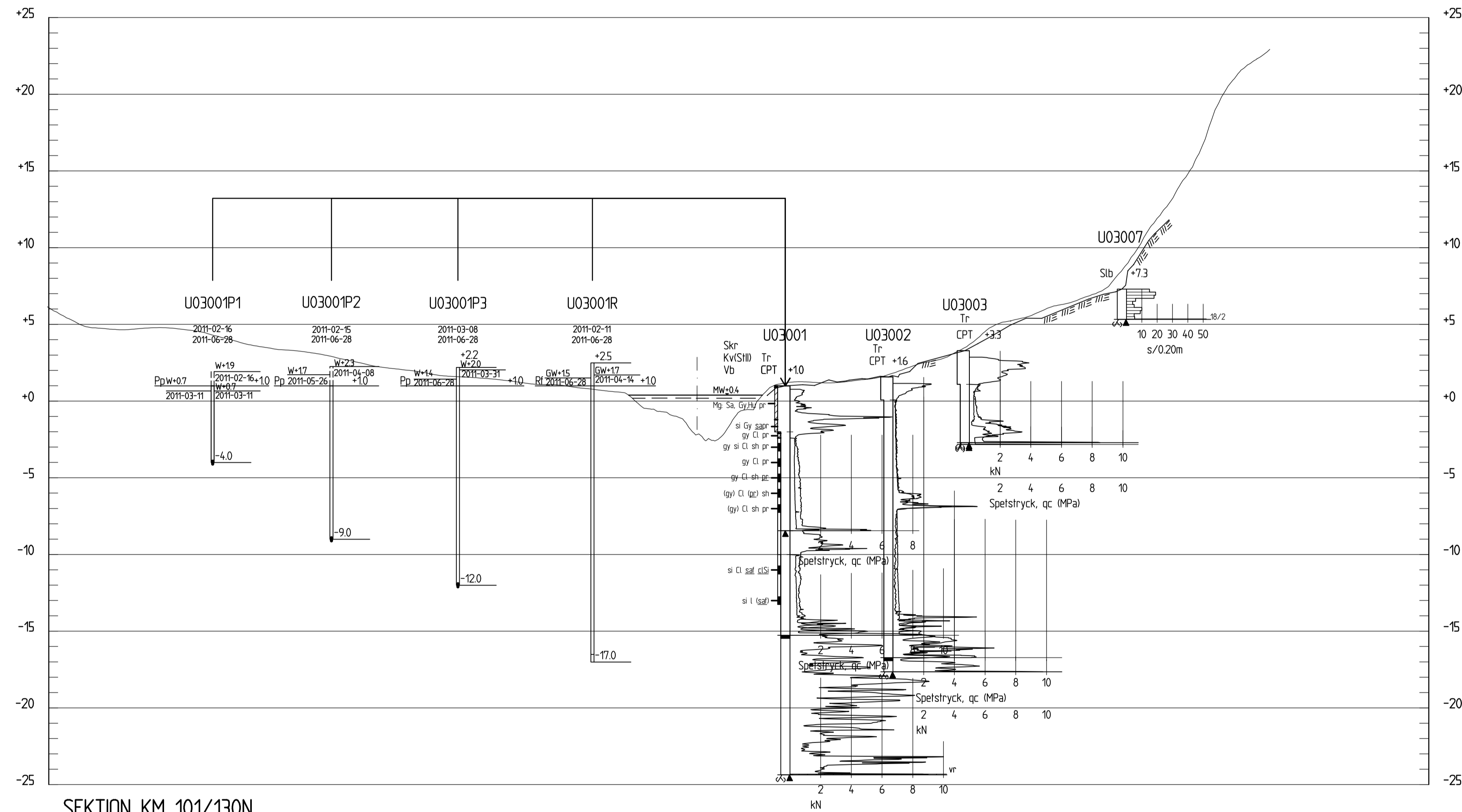
SEKTION KM 101/130N H 1:200 L 1:1000
