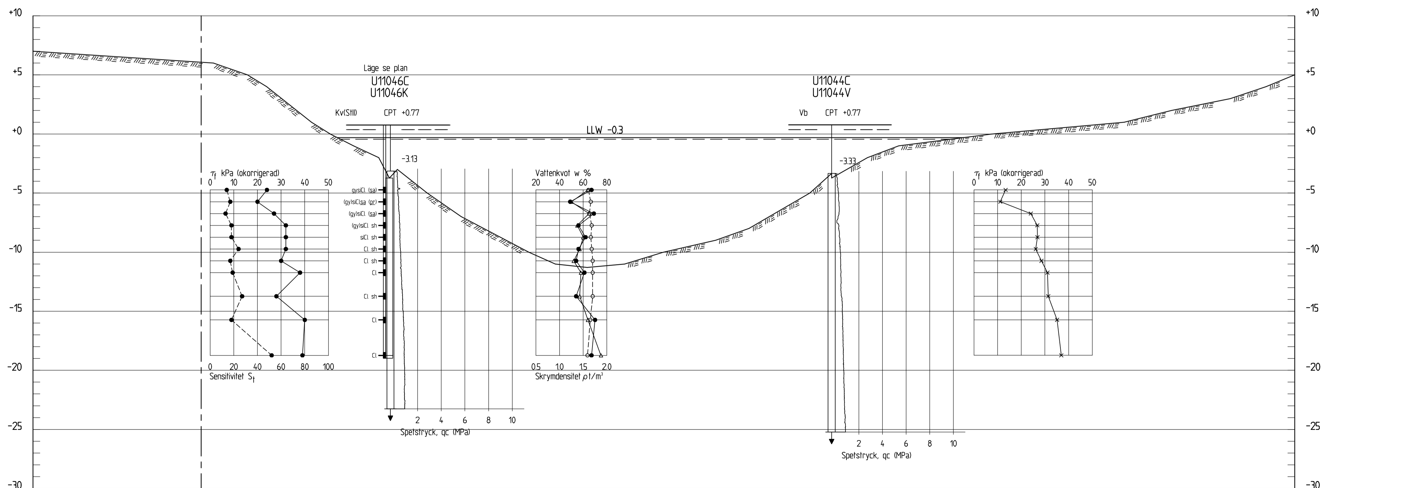
SEKTION 37/900 H 1: 200 L 1: 400
