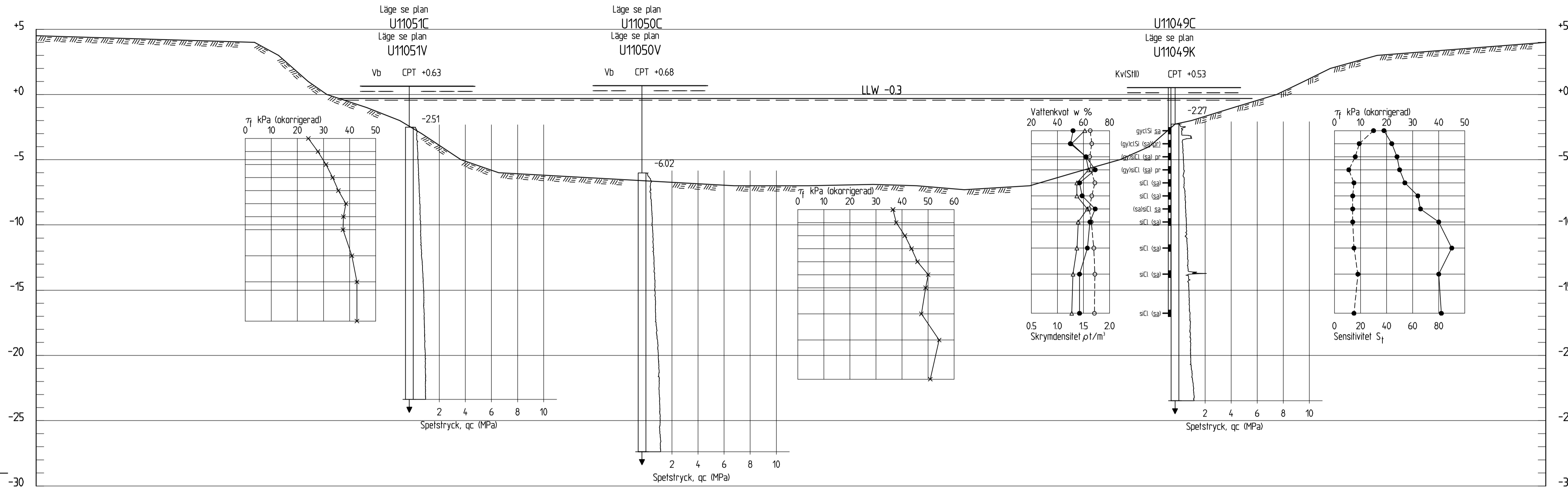
SEKTION 41/200 H 1:200 L 1:500
