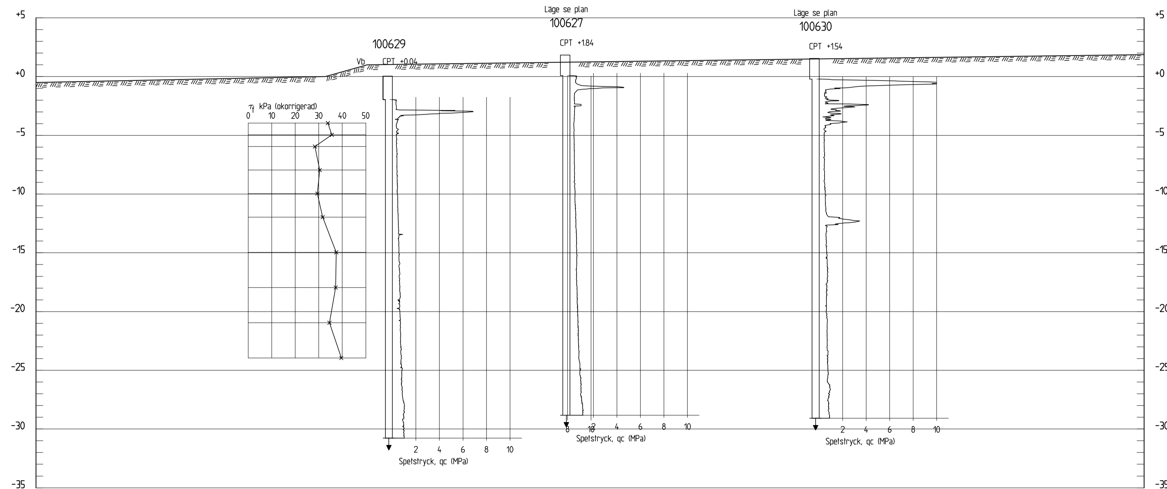
SEKTION 81/700 - 81/825 H 1: 200 L 1: 400
