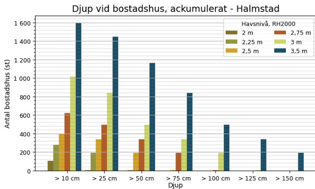
Figur 13 Samband i Halmstad kommun mellan havsnivå och antalet bostadshus som översvämmas med ett givet vattendjup eller mer. Förutsätter att havsnivån varar tillräckligt länge för att maximalt potentiellt översvämningsdjup ska hinna nås.
