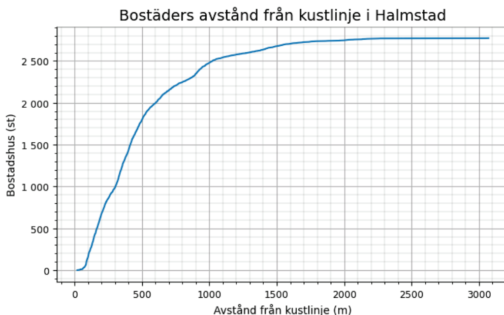
Figur 16 Antal bostadshus på givet avstånd från kusten som översvämmas vid havsnivåer <5 m (RH2000) i Halmstad kommun. X-axelns utbredning bestäms av det maximala avståndet från kustlinjen till ett bostadshus som översvämmas vid <5 m (RH2000).
