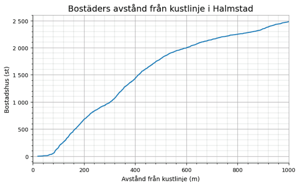
Figur 17 Antal bostadshus inom 1 km från kusten som översvämmas vid havsnivåer <5 m (RH2000) i Halmstad kommun.
