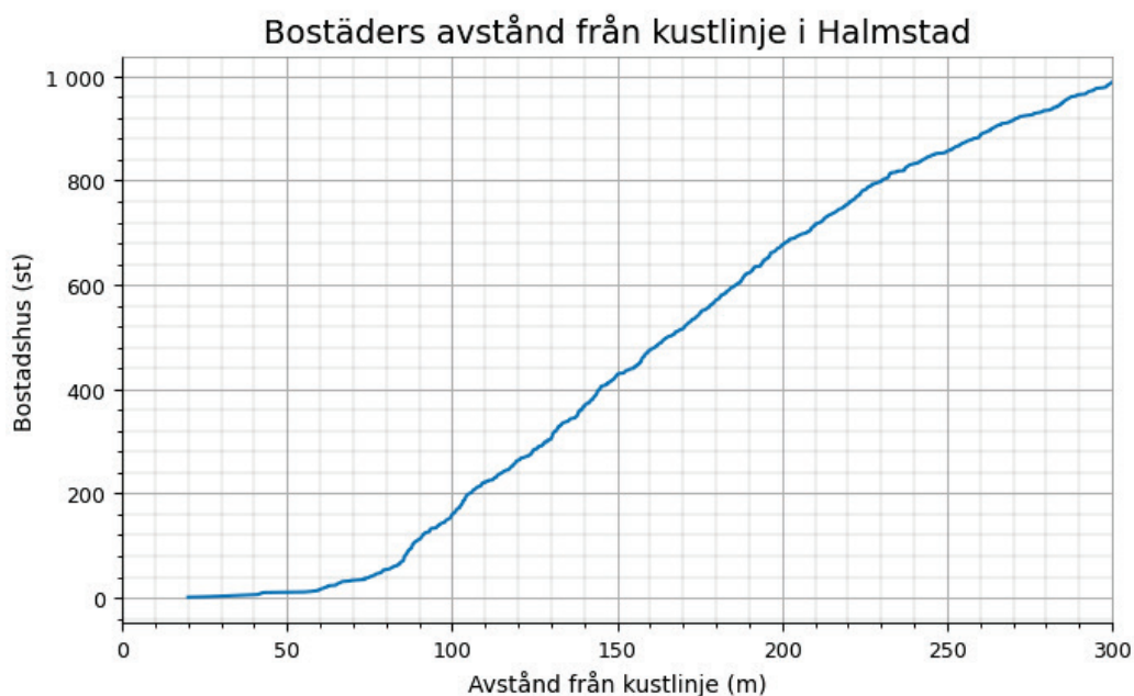
Figur 18 Antal bostadshus inom 300 m från kusten som översvämmas vid havsnivåer <5 m (RH2000) i Halmstad kommun.
