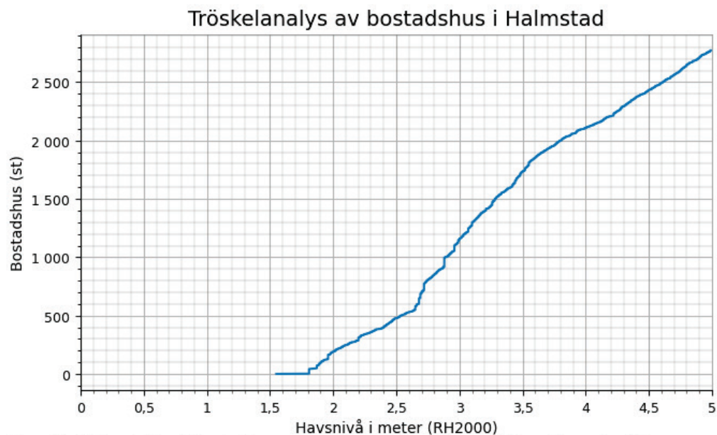
Figur 4 Antalet bostadshus i Halmstad kommun som riskerar att översvämmas vid havsnivåer mellan 0-5 m. Bostadshus kan delas in i följande ändamål: Småhus friliggande, Småhus kedjehus, Småhus radhus, Småhus med flera lägenheter och Flerfamiljshus.
