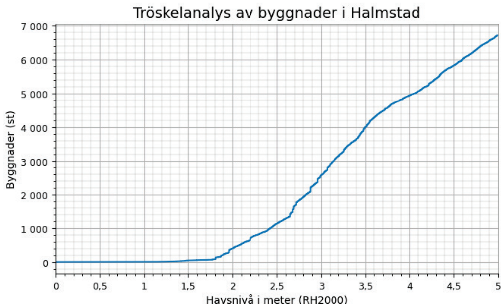
Figur 3 Antalet byggnader i Halmstad kommun som riskerar att översvämmas vid havsnivåer mellan 0-5 m. Byggnader består av följande objektstyper: Bostad, Industri, Samhällsfunktion, Verksamhet, Ekonomibyggnad, Komplementbyggnad och Övrig byggnad.
