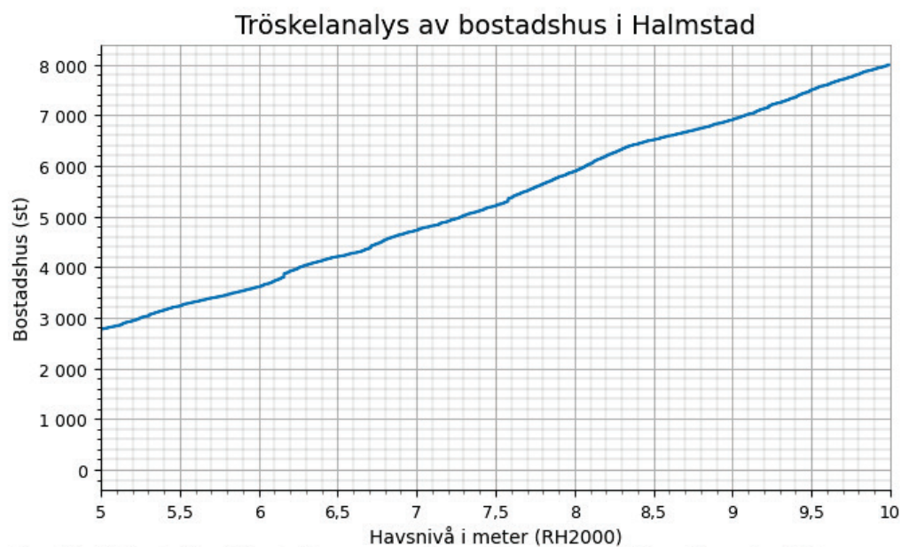
Figur 5 Antalet bostadshus i Halmstad kommun som riskerar att översvämmas vid havsnivåer mellan 5-10 m. Bostadshus kan delas in i följande ändamål: Småhus friliggande, Småhus kedjehus, Småhus radhus, Småhus med flera lägenheter och Flerfamiljshus.
