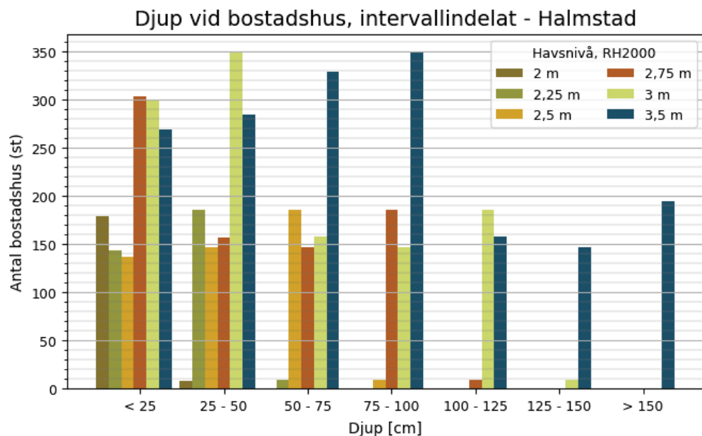
Figur 12 Samband i Halmstad kommun mellan havsnivå och antalet bostadshus som drabbas av översvämning, indelat i intervall för översvämningsdjup vid bostad. Förutsätter att havsnivån varar tillräckligt länge för att maximalt potentiellt översvämningsdjup ska nås.
