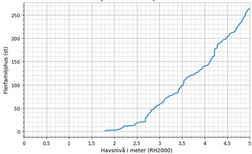
Figur 6 Antalet flerfamiljshus i Halmstad kommun som riskerar att översvämmas vid havsnivåer mellan 0-5 m.
