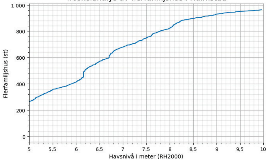
Figur 7 Antalet flerfamiljshus i Halmstad kommun som riskerar att översvämmas vid havsnivåer mellan 5-10 m.
