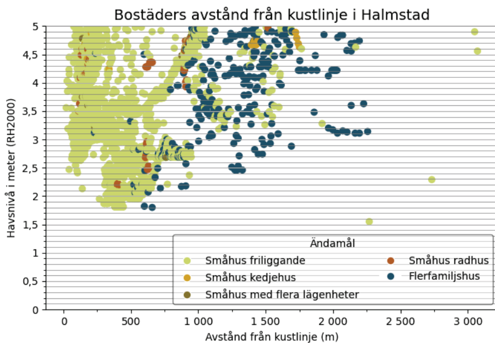
Figur 19 Samband mellan tröskelnivå för havsöversvämning, avstånd från kustlinjen och ändamålet för bostadshus i Halmstad kommun. X-axelns utbredning bestäms av det maximala avståndet från kust till ett bostadshus som översvämmas vid <5 m (RH2000).
