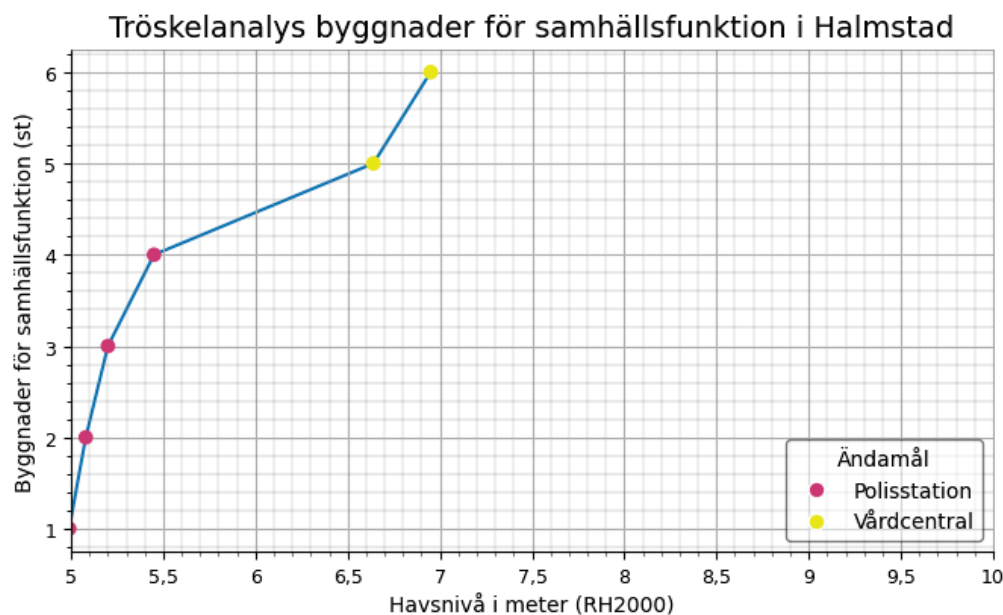
Figur 9 Antal byggnader för samhällsfunktion i Halmstad kommun som riskerar att översvämmas vid havsnivåer mellan 5-10 m. De samhällsfunktioner som inkluderas i analysen är Sjukhus, Brandstation, Vårdcentral, Kommunhus och Polisstation.
